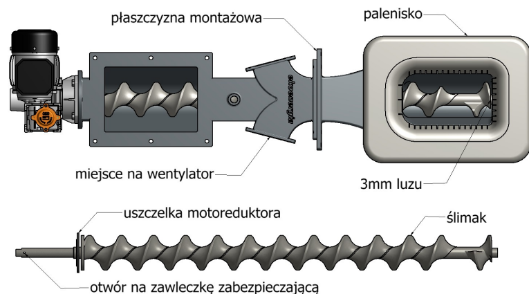
Rysunek 1. Schemat montażowy wielopaliwowego palnika retortowego.
